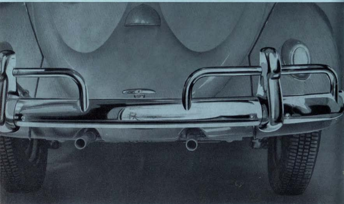
No. 855 Rammschutz vorne und hinten, verchromt, kompletter Satz – Pare-chocs supplémentaires, avant et arrière, chromés, jeu complet
